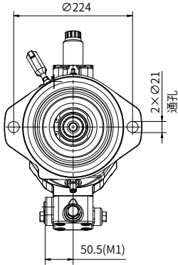
X向视图
