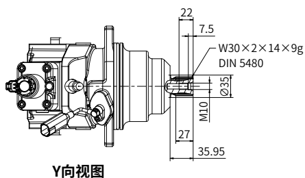
Y向视图
