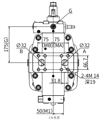
Z向视图
