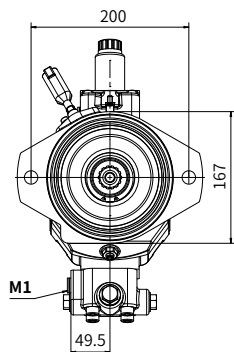
X向视图
