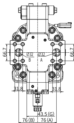
Z向视图
