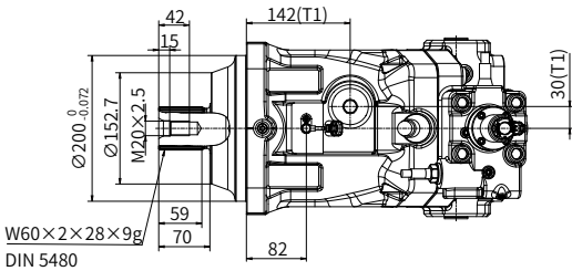
Y向视图
