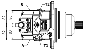
Y向视图
