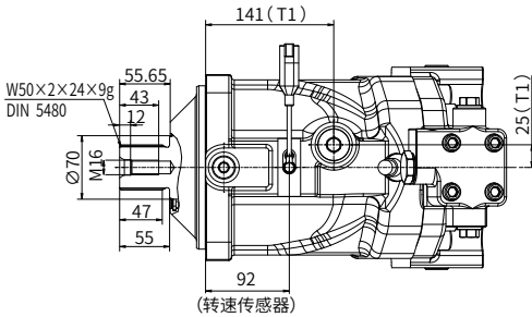
Y向视图
