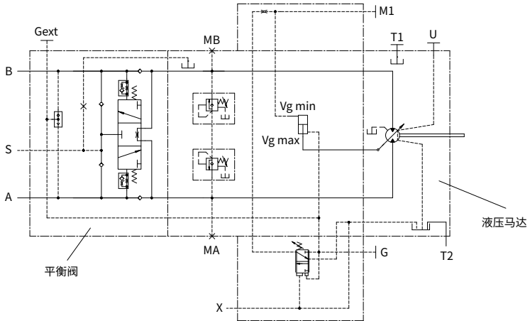
平衡阀
