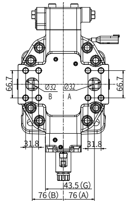
Z向视图
