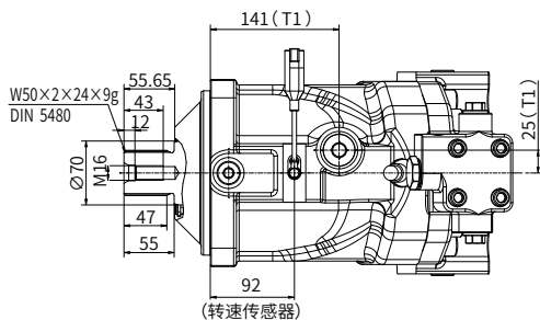
Y向视图
