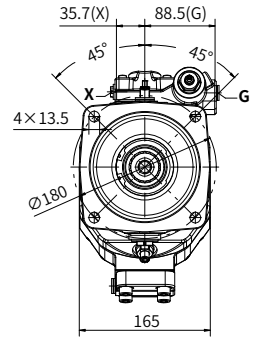
X向视图
