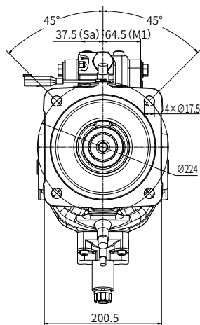
X向视图
