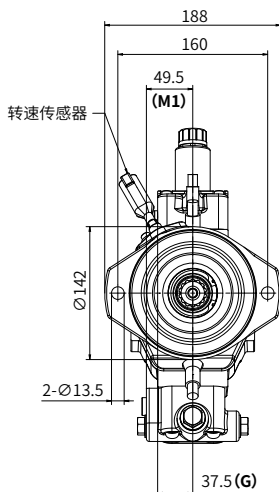
X向视图
