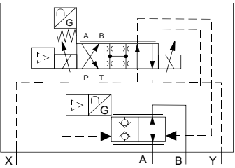
2WRCE..-L2X/P...L...
