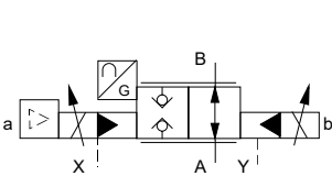
2WRCE..-L2X/P...L...
