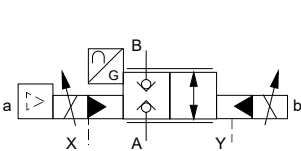
2WRCE..-L2X/P...
