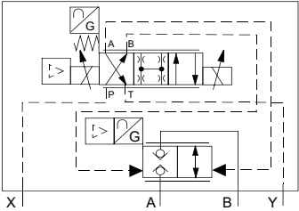
2WRCE..-L2X/P...
