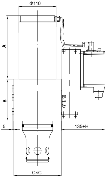
通径 50
